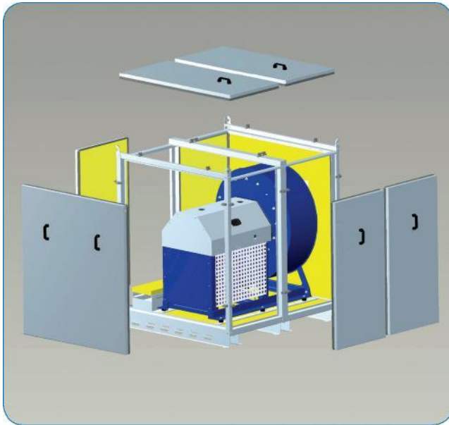
Klemmbügel an den Bauteilen ermöglichen einen schnellen Zutritt.
